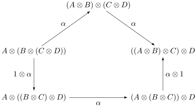
(“Mac Lane’s pentagon”)
