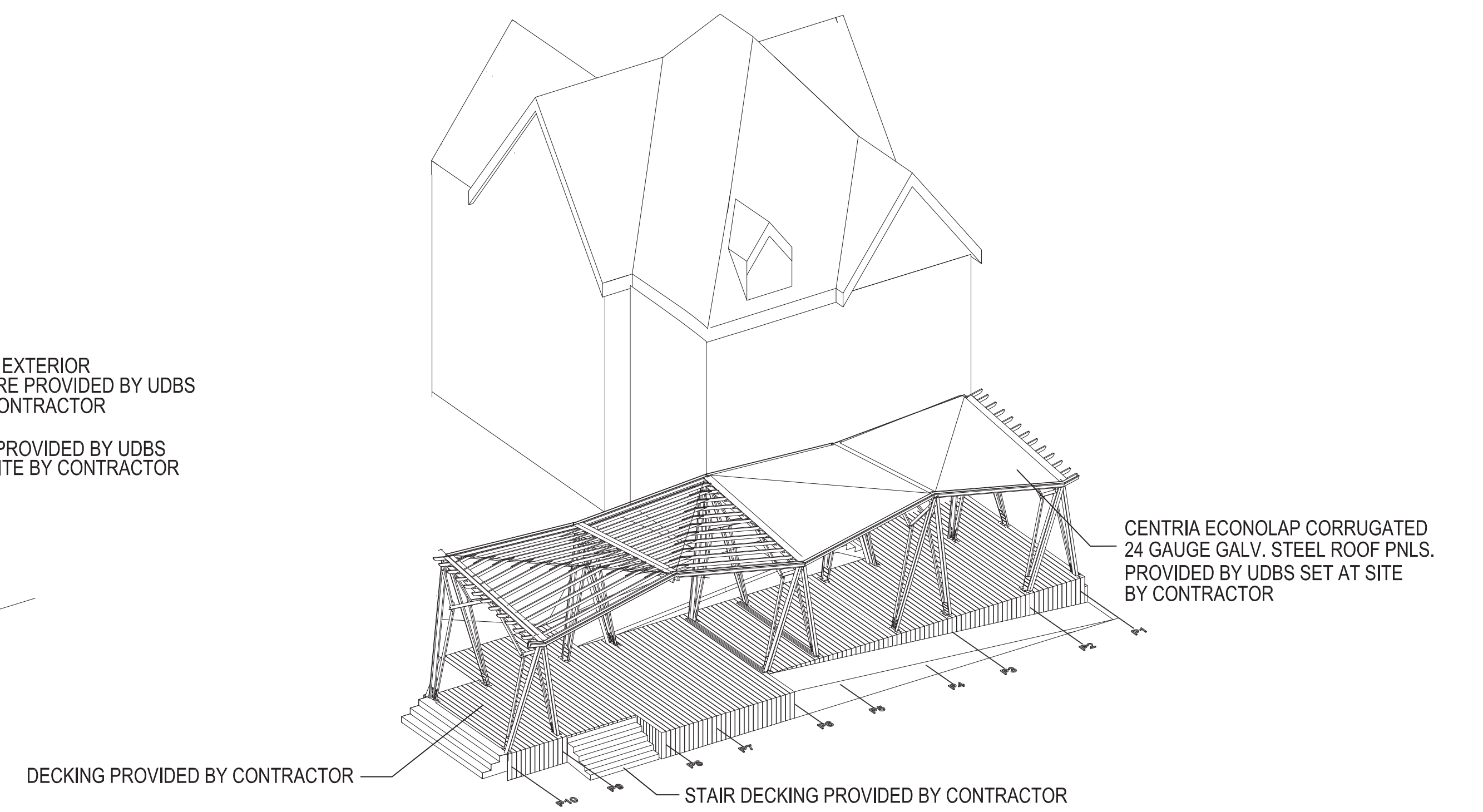
15 METAL SHEETING BAY 01-02 N.T.S.
