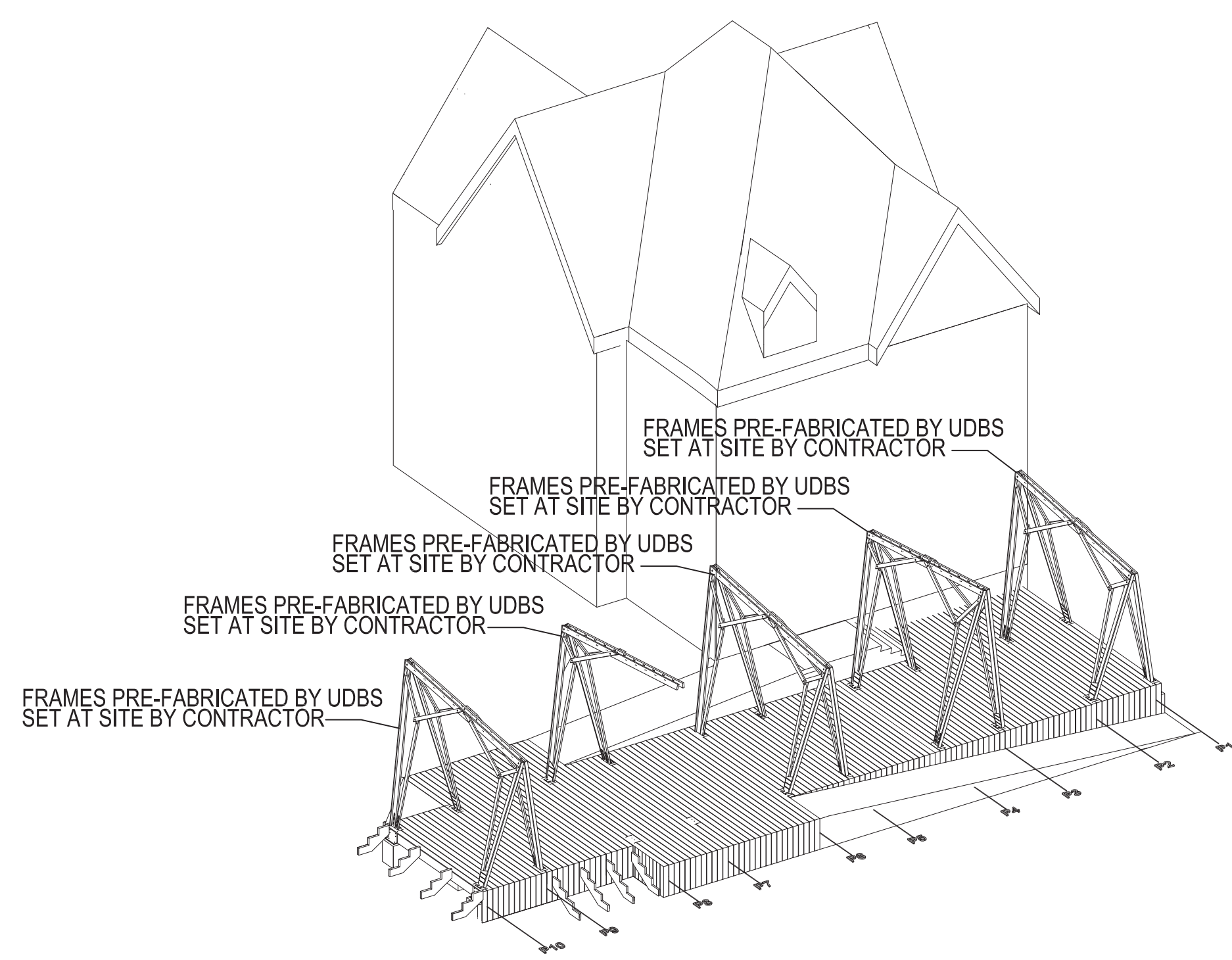
10 DECKING N.T.S.
