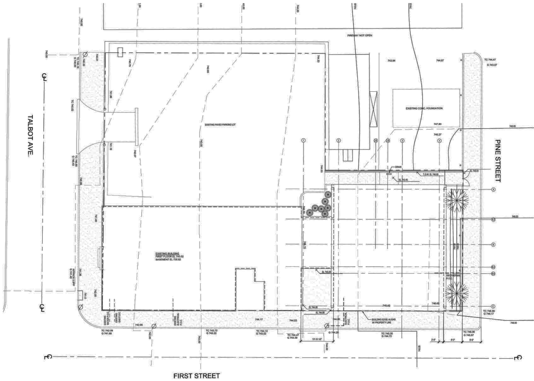
A2 SITE PLAN SCALE: 1/8" = 1'-0"
