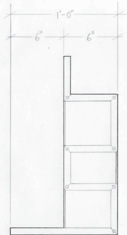
RIGHT ELEVATION
